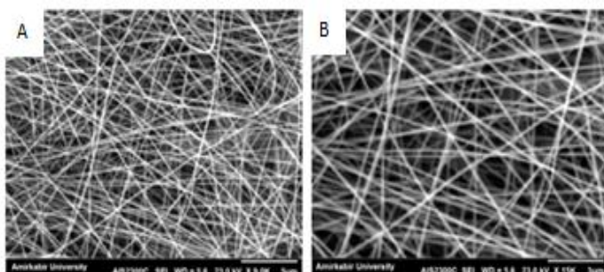
شکل ۱. تصویر نانو داربست PCL-Gelatin ساخته شده به روش الکتروریسی، تصویر برداری توسط میکروسکوپ الکترونی اسکنینگ (مدل S-416 FESEM) در ولتاژ ۱۵ کیلو ولت.
