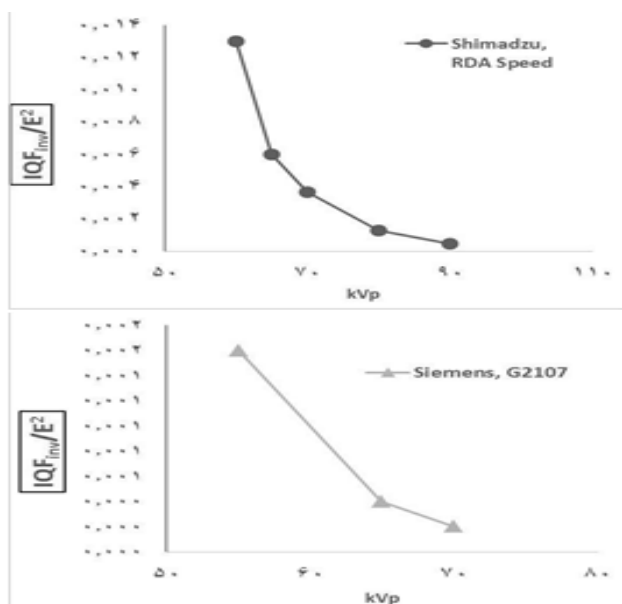
نمودار ۲. نمودار IQF_{Inv}/E^2 برحسب kVp برای Shimadzu, RDA Speed در فاصله چشمه تا آشکارساز ۱۵۰ سانتیمتر و Siemens, G2107 در فاصله چشمه تا آشکارساز ۱۱۰ سانتیمتر
