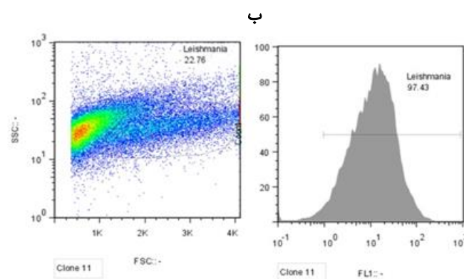
شکل ۴. الف) تصویر انگل L. tropica EGFP-LUC با استفاده از میکروسکوپ فلورسنت (درشتنمایی ×۱۰۰۰). ب) نتایج شدت فلورسنت EGFP در انگل L. tropica EGFP-LUC با استفاده از فلوسایتومتري
