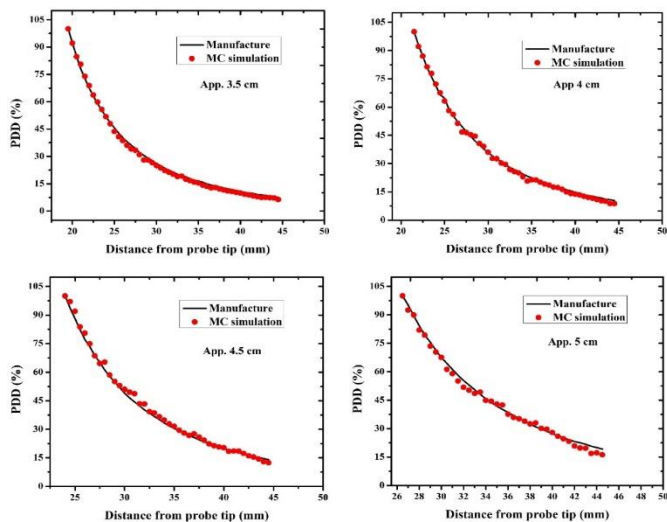
شکل ۴. مقایسه منحنی‌های PDD حاصل از شبیه‌سازی مونت کارلو و نتایج گزارش شده توسط شرکت سازنده برای اپلیکاتورهای کروی با قطر ۳/۵ cm تا ۵ cm
