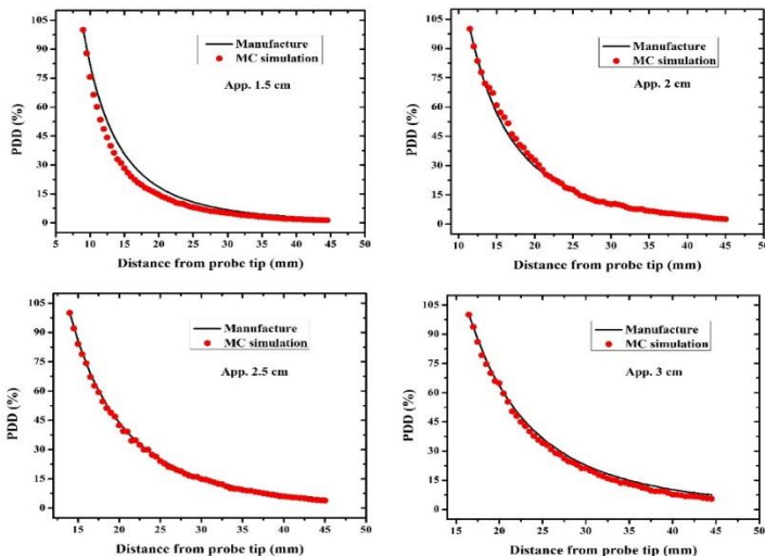
شکل ۳. مقایسه منحنی‌های PDD حاصل از شبیه‌سازی مونت کارلو و نتایج گزارش شده توسط شرکت سازنده برای اپلیکاتورهای کروی با قطر ۱/۵ cm تا ۳ cm
