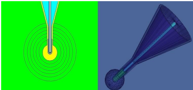
شکل ۱. نمای دوبعدی و سه‌بعدی از پروب اشعه ایکس و اپلیکاتور ۲/۵ cm که توسط کد MCNPX شبیه‌سازی شده است. فضای اطراف اپلیکاتور به سطوح کروی هم‌مرکز تقسیم شده تا بتوان از تکنیک کاهش‌وریانس تقسیم‌هندسه و رولت روسی استفاده کرد.
