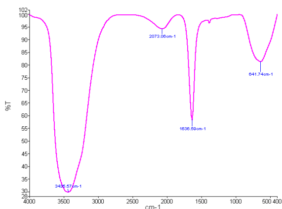
شکل ۳. طیف سنجی مادون قرمز (FTIR) نانوذرات نقره سنتز شده. باند های جذبی در نواحی 2073 \text{ cm}^{-1} و 2048 \text{ cm}^{-1} مربوط به ترکیبات آلکین ستون و باند 1630 \text{ cm}^{-1} مربوط به آلکن ها است که می تواند بر اثر واکنش با عصاره گیاهی ایجاد شده باشد. باند جذبی 3435 \text{ cm}^{-1} مربوط به ترکیبات هیدروکسیدی مربوط به عصاره گیاهی با نانوذرات نقره بوده است.
