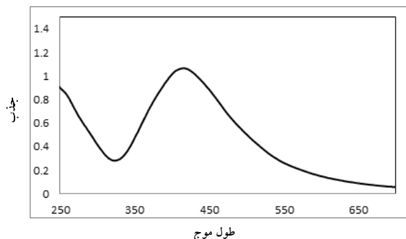
شکل ۱. طیف سنجی UV-Vis نانوذرات نقره سنتز شده. با توجه به نمودار، ماکزیم جذب UV نانوذرات نقره در طول موج 438 \text{ nm} نانومتر می باشد. نتایج تفرق اشعه ایکس (XRD) نانوذرات نقره
