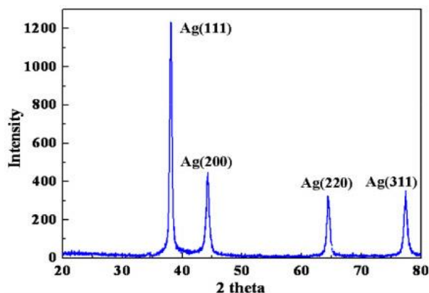
شکل ۲ ب. طیف نمونه استاندارد نانوکریستال های نقره.
