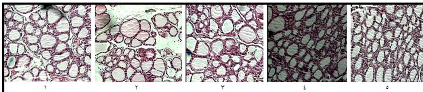
شکل ۱. فتومیکروگراف نوری از بافت تیروئید در گروه (۱) کنترل، (۲) شش، (۳، ۴ و ۵) گروه های دریافت کننده دوز ۵۰، ۱۰۰ و ۲۰۰ mg/kg عصاره هیدروالکلی گیاه پنج انگشت با رنگ آمیزی هماتوکسیلین-انوزین و با بزرگنمایی ۱۰۰×
