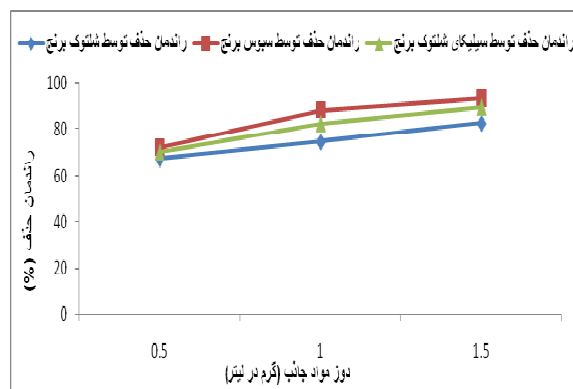
نمودار ۳. اثر جرم جاذبههای شلتوک، سیوس و سیلیکای حاصل از شلتوک برنج بر راندمان حذف کادمیوم در pH ۶ غلظت اولیه کادمیوم ۵ میلی گرم در لیتر و زمان تماس ۶۰ دقیقه
