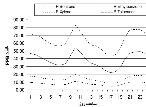
شکل ۴. میانگین غلظت به دست آمده برای ساعات مختلف روز برای چهار آلایند بنزن، تولوئن، اتیل بنزن و زایلین در ایستگاه شهر ری
