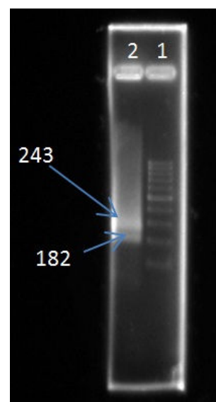
شکل ۱. الکتروفورز برش محصول PCR مربوط به ناحیه کربوکسیل انتهایی پروتئین PA با سبیل سیاه زخم روی ژل آگارز ۲ درصد. ۱. DNA ladder و ۲. باندهای ۱۸۲ و ۲۴۳ حاصل از برش آنزیمی توسط Eco57I (AclI)
