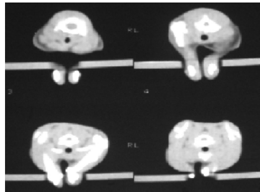
شکل ۲. مقاطع CT جهت تعیین عمق نخاع
