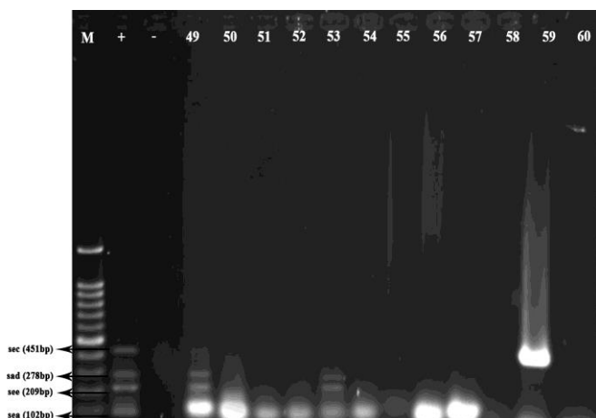
شکل ۳. واکنش M-PCR برای شناسایی ژن های انتروتوکسین استافیلوکوک اورئوس ستون M: سایز مارکر ۱۰۰bp، کنترل مثبت واجد ژن sea (۱۰۲bp)، ژن see (۲۰۹bp)، ژن sec (۴۵۱bp)، ژن sed (۲۷۸bp)، کنترل منفی (استافیلوکوک اپیدرمیدیس)، نمونه ۵۱، ۵۲، ۵۳، ۵۴، ۵۵، ۵۶، ۵۷ واجد ژن sea، نمونه های ۴۹ و ۵۳ واجد ژن see، نمونه های ۴۹ و ۵۳ واجد ژن sed، نمونه ۵۹ واجد ژن sec
