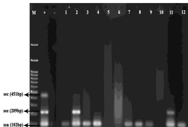
شکل ۲. واکنش M-PCR برای شناسایی ژن های انتروتوکسین استافیلوکوک اورئوس ستون M: سایز مارکر ۱۰۰bp، کنترل مثبت واجد ژن sea (۱۰۲bp)، ژن see (۲۰۹bp)، ژن sec (۴۵۱bp)، ژن sed (۲۷۸bp)، کنترل منفی (استافیلوکوک اپیدرمیدیس)، نمونه ۴۷ واجد ژن see، نمونه های ۳۶، ۳۷، ۳۸ و ۳۹ واجد ژن sed
