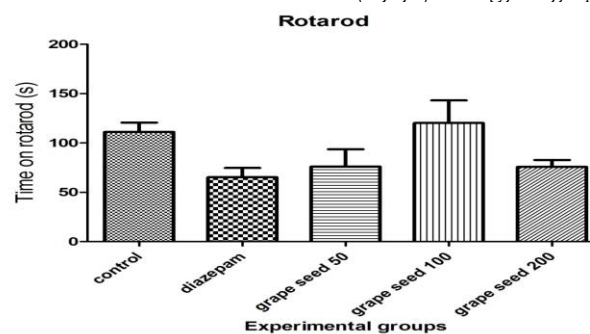
نمودار ۳. مقایسه تعادل حرکتی در گروههای آزمایشی
